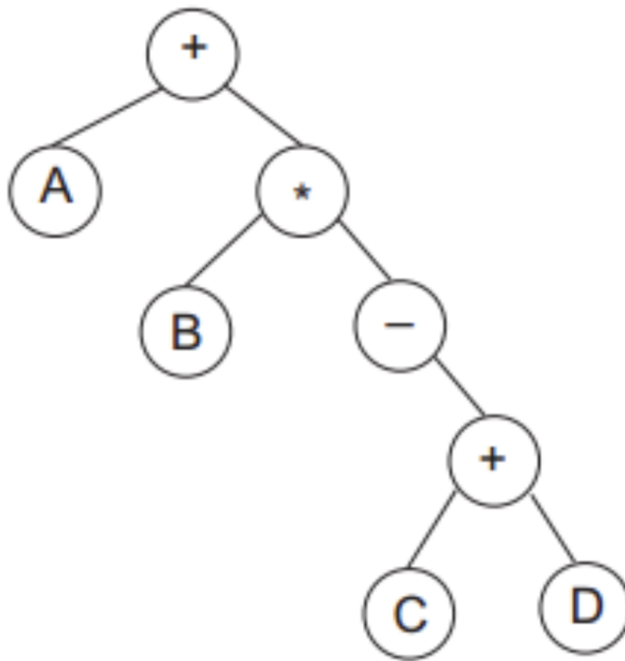
Figura 16: Ejemplo de árbol de expresión #4
