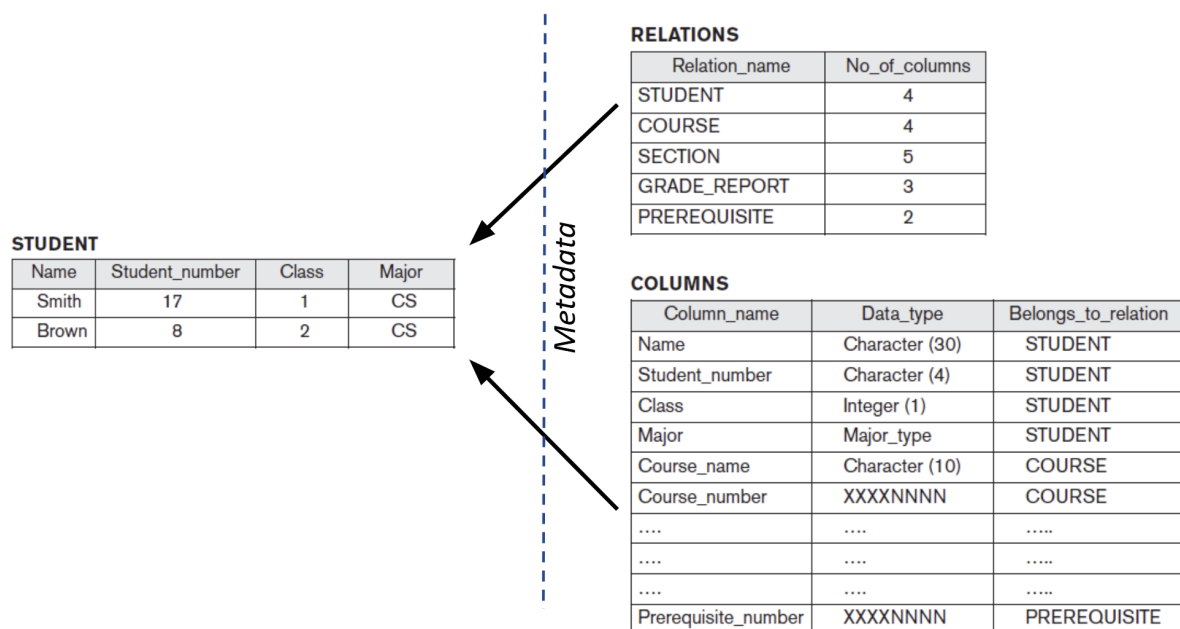
Figura 111: Metadata en los DBMS
