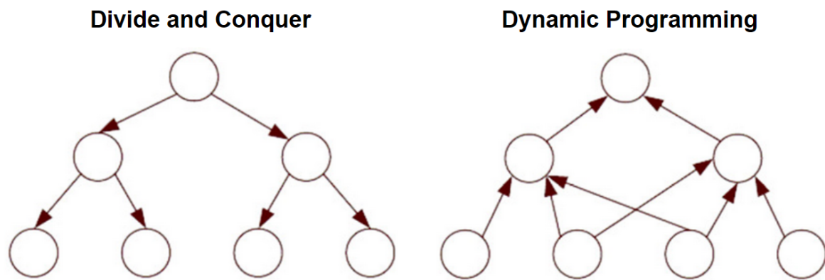
Figura 96: Divide y conquista vs programación dinámica
