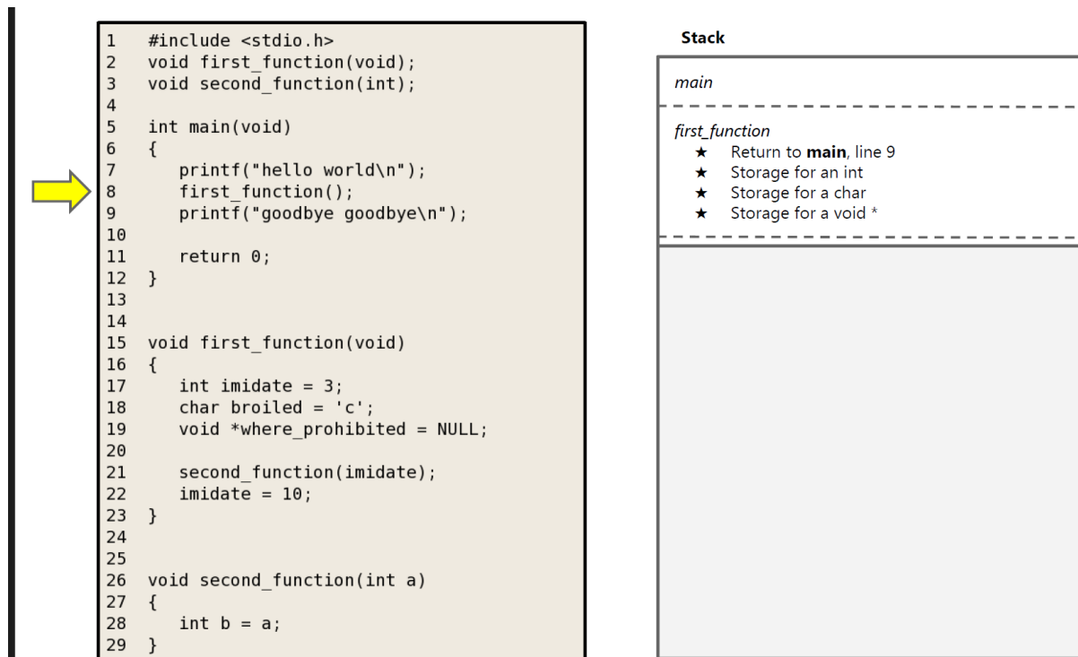
Figura 75: Visualización del stack (2 de 5)
