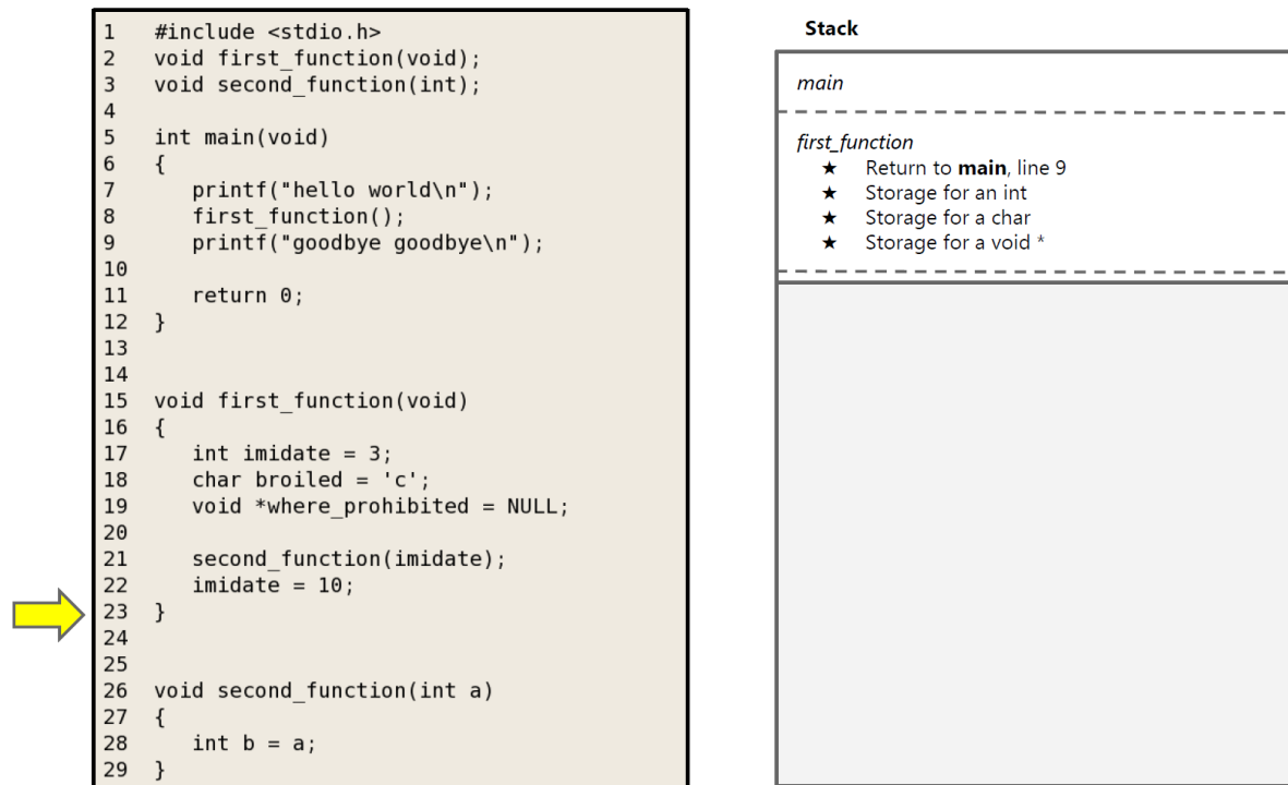
Figura 77: Visualización del stack (4 de 5)
