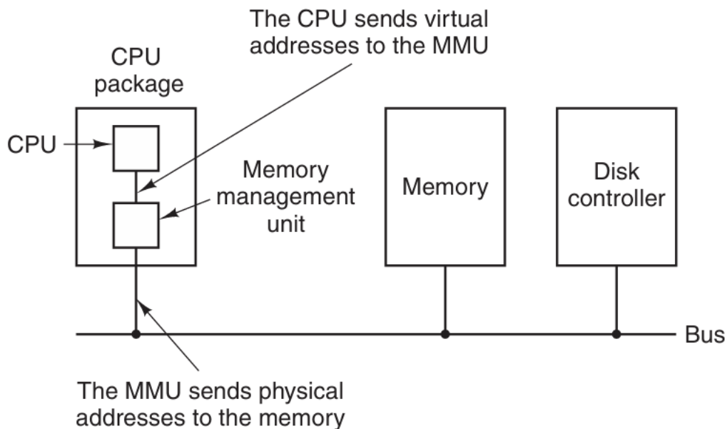
Figura 72: Relación entre direcciones virtuales y físicas
