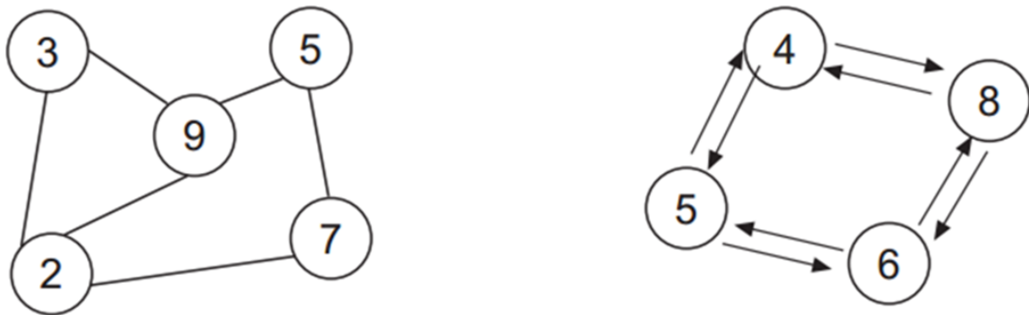
Figura 50: grafo conexo y fuertemente conexo
