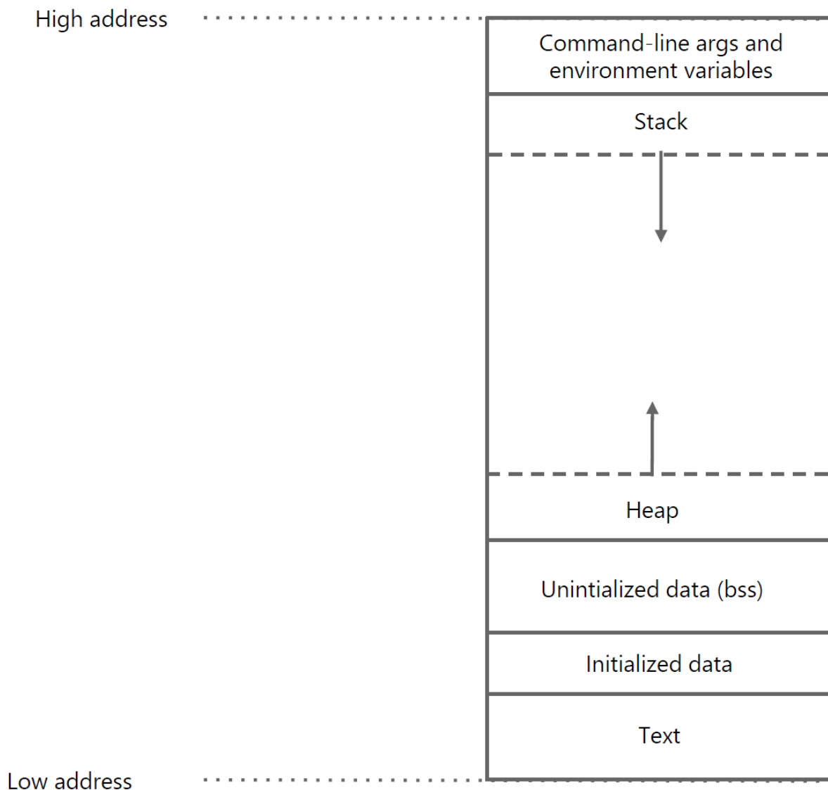
Figura 73: Layout de memoria de un programa en C
