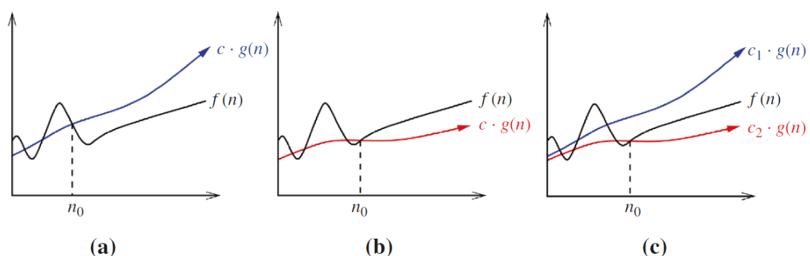
Figura 90: Visualización de Big O, Big Omega y Big Theta
