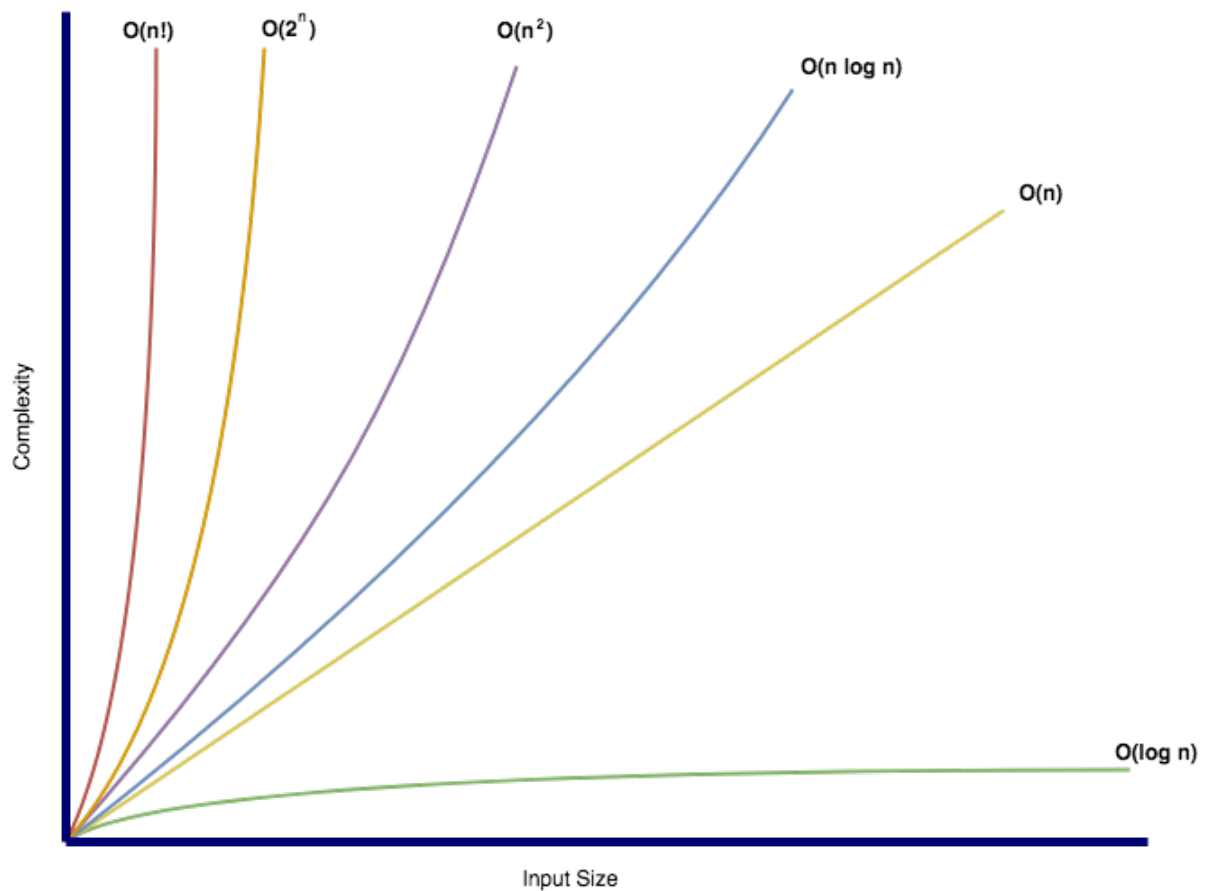
Figura 91: Gráfico de Big-O conocidas
